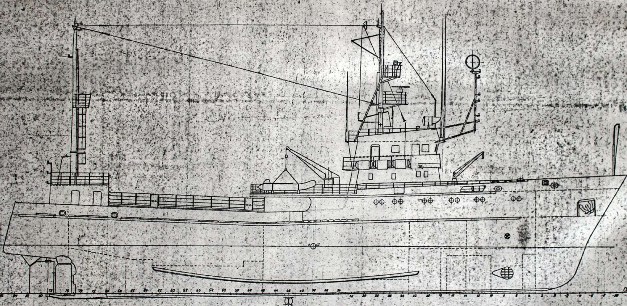
Боковой вид
