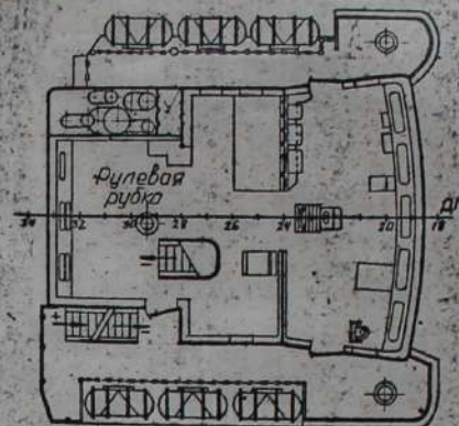
Ходовой мостик
