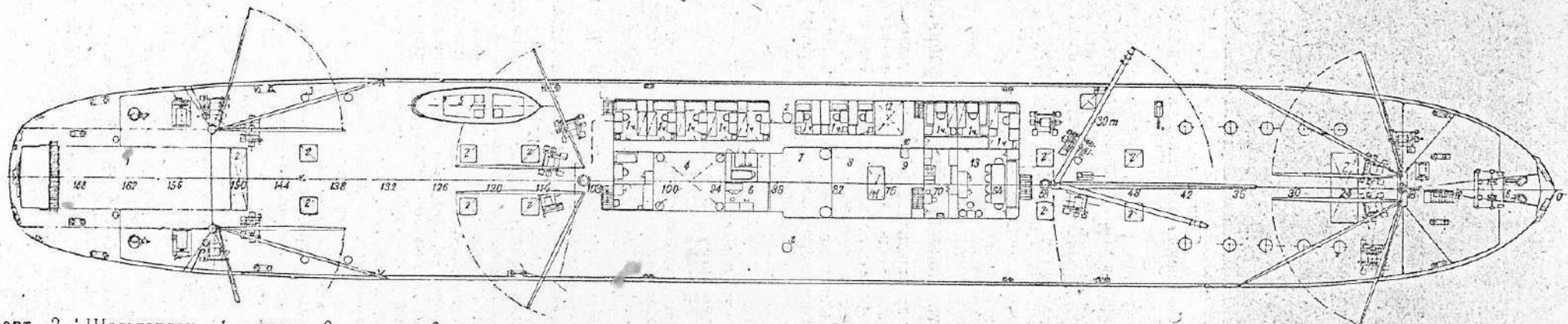
Черт. 2. Шельтердек. 1 — слип; 2 — люки; 3 — горловины к аппаратам „Рюгнер Вгух“; 4 — машинная шахта; 5 — буксирный катер; 6 — лаборатория; 7 — котельная шахта; 8 — камбуз; 9 — хлебопекарня; 10 — элеватор; 11 — люк для погрузки угля; 12 — углехранилище для китобойцев; 13 — кают-компания.
