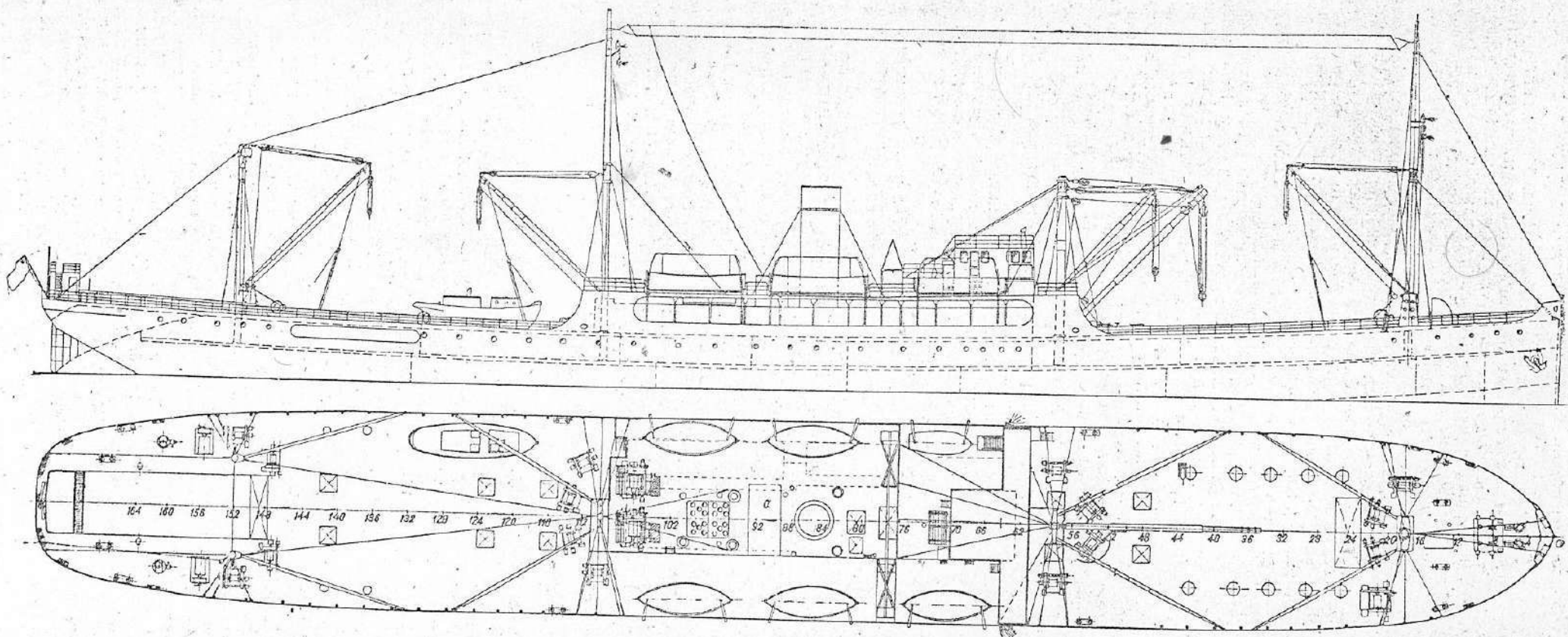
Черт. 1. Боковой вид и вид сверху. а — радиорубка.
