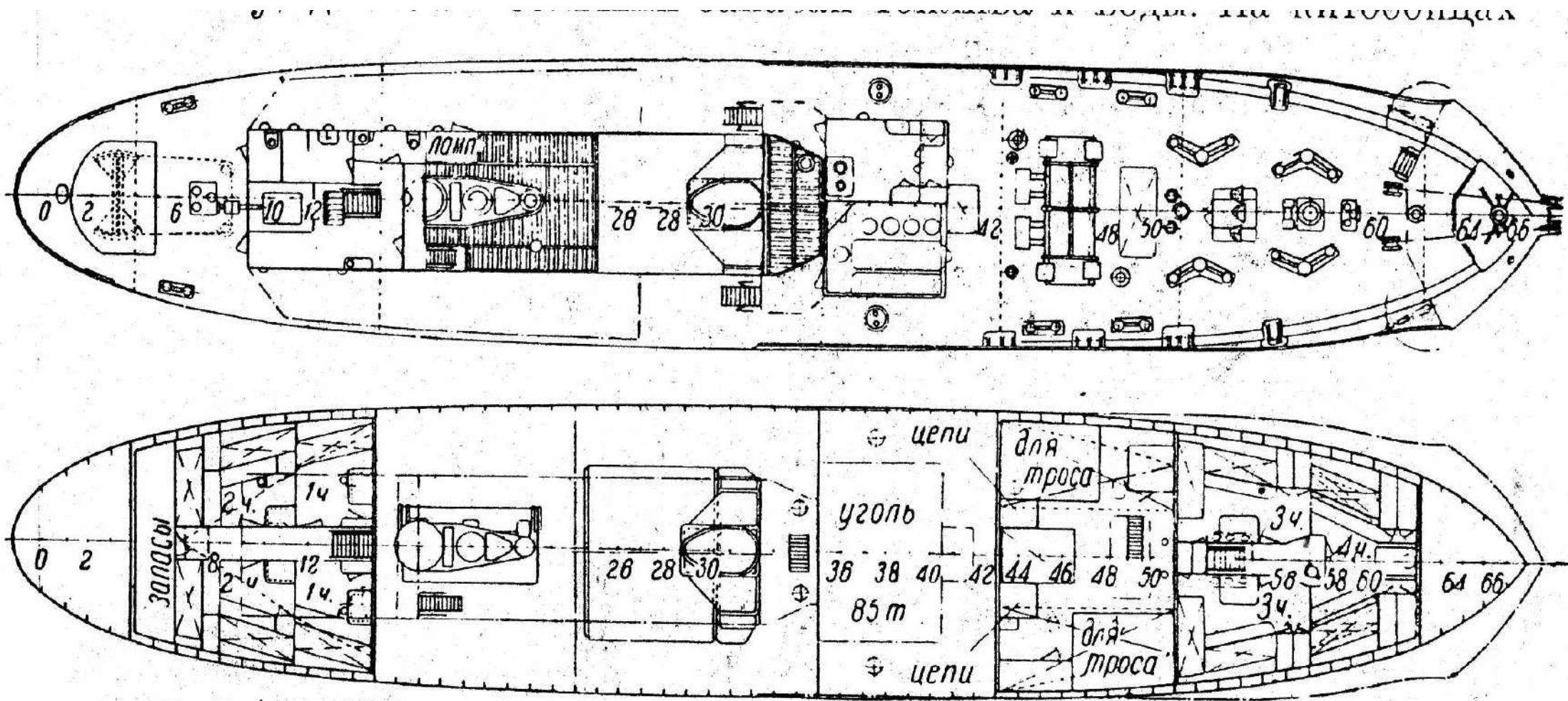
Фиг. 30. Советское китобойное судно. Палубы и трюм.
