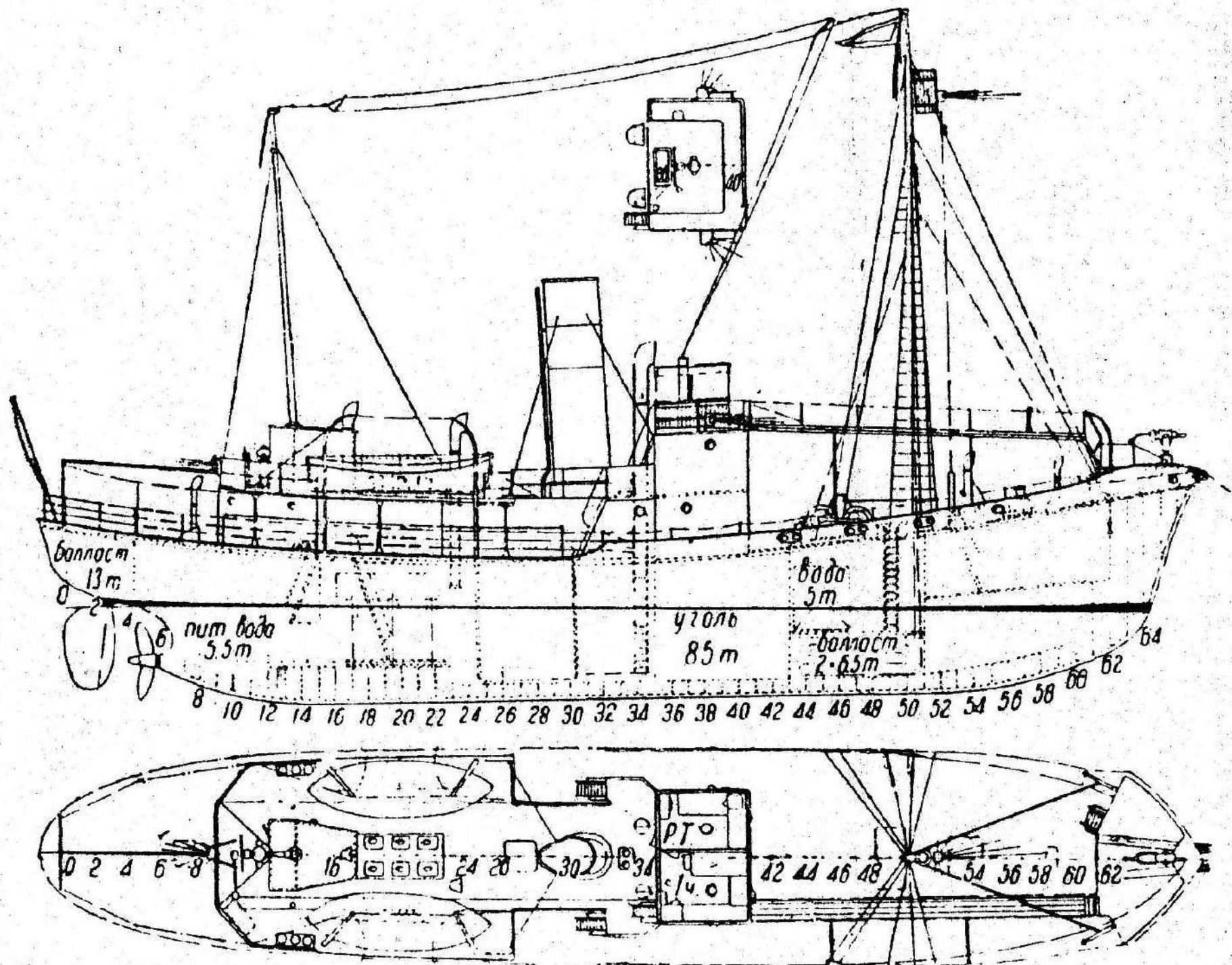
Фиг. 29. Советское китобойное судно. Боковой вид и надстройки.
