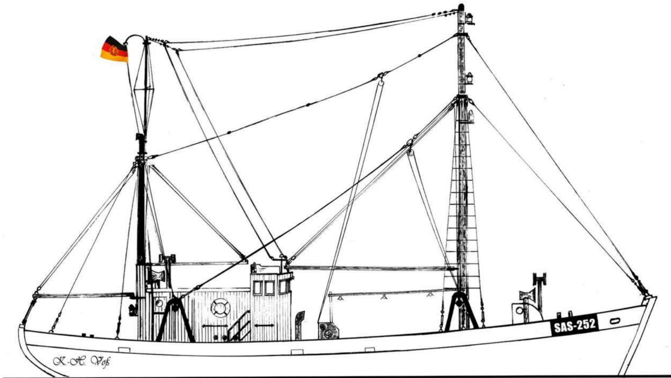
Damgartener Kutter · Zeichnung: K.-H. Voß
