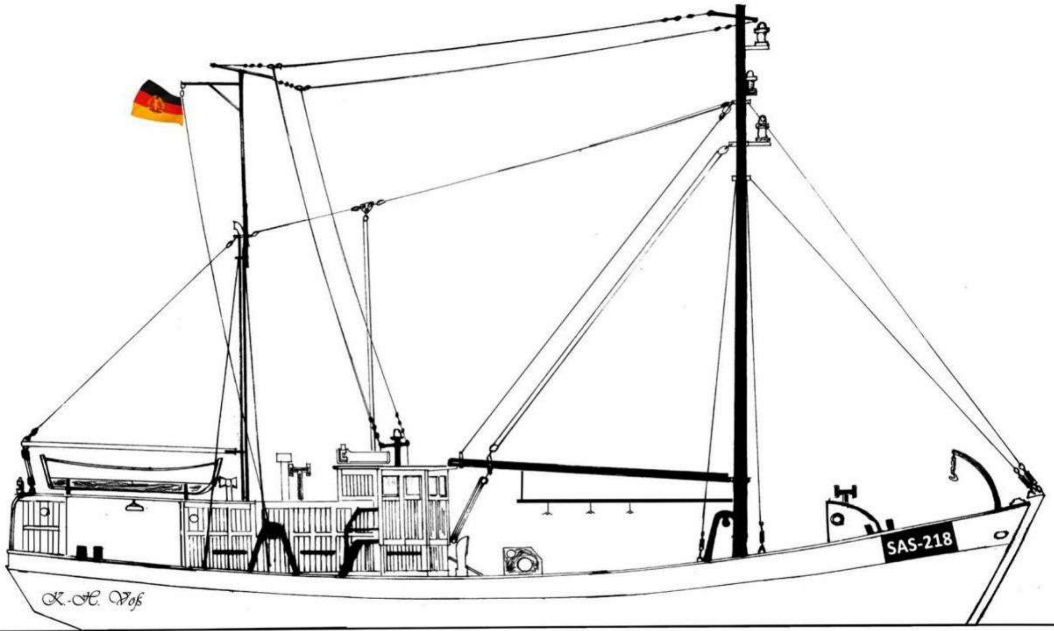
Gehlsdorfer Kutter · Zeichnung: K.-H. Voß
