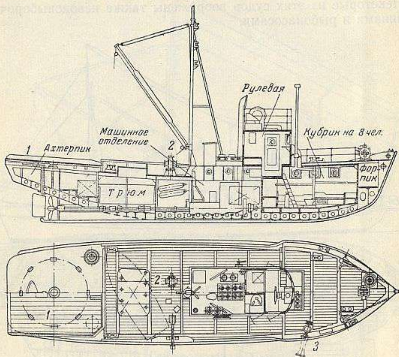
Рис. 12. Малый рыболовный сейнер
