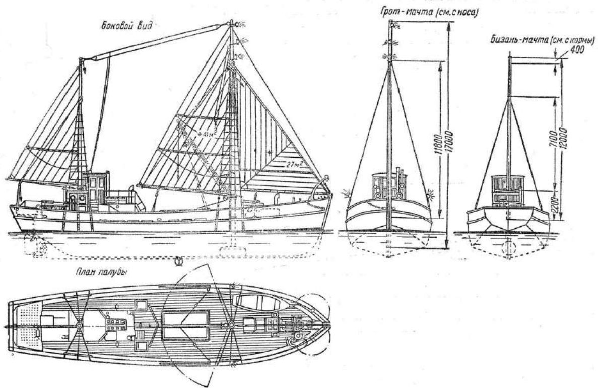
Рис. 340. Малый дрейфтер-сейнер для Каспийского моря. Общий вид (элементы см. табл. 73—15).
