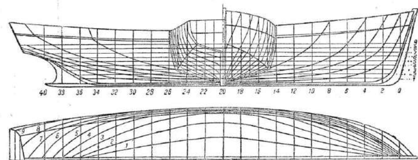
Рис. 341. Малый дрейфтер-сейнер. Теоретический чертеж.
