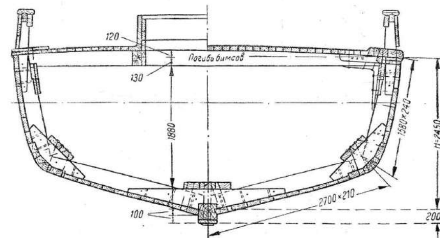
Рис. 342. Малый дрейфтер-сейнер. Поперечное сечение.
