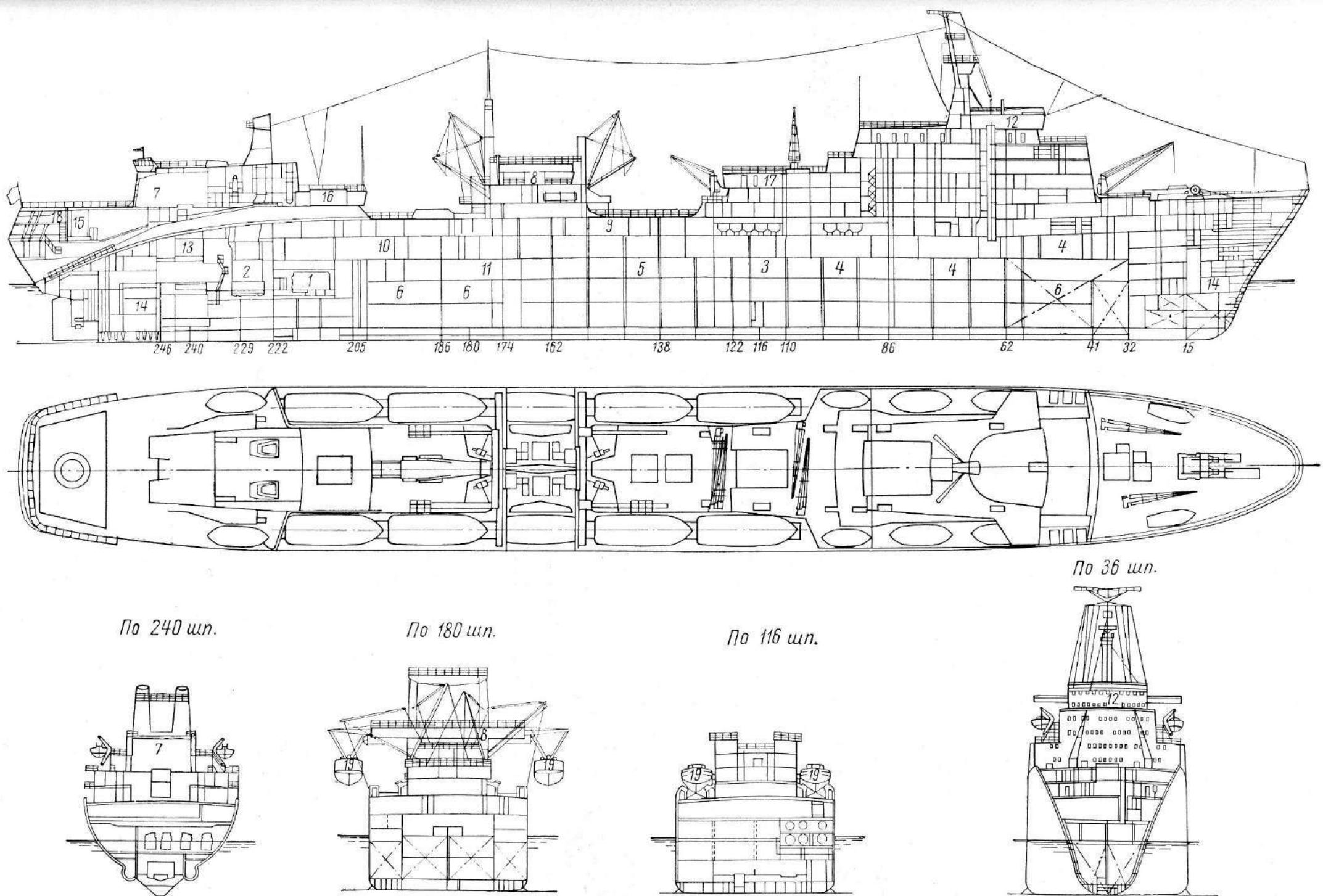
Рис. 1. Продольный разрез, план палубы и поперечные сечения базы.
