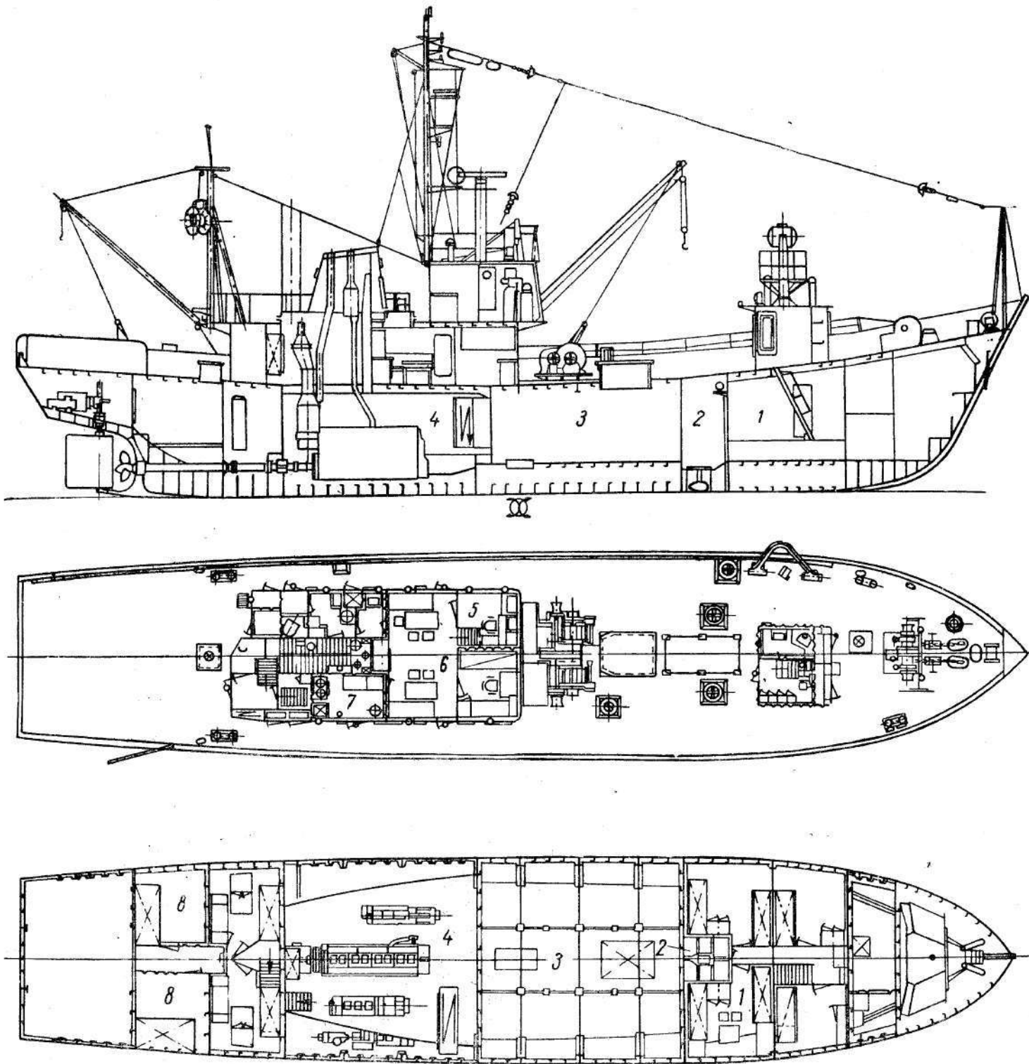
Рис. 2. Общее расположение сейнера.
