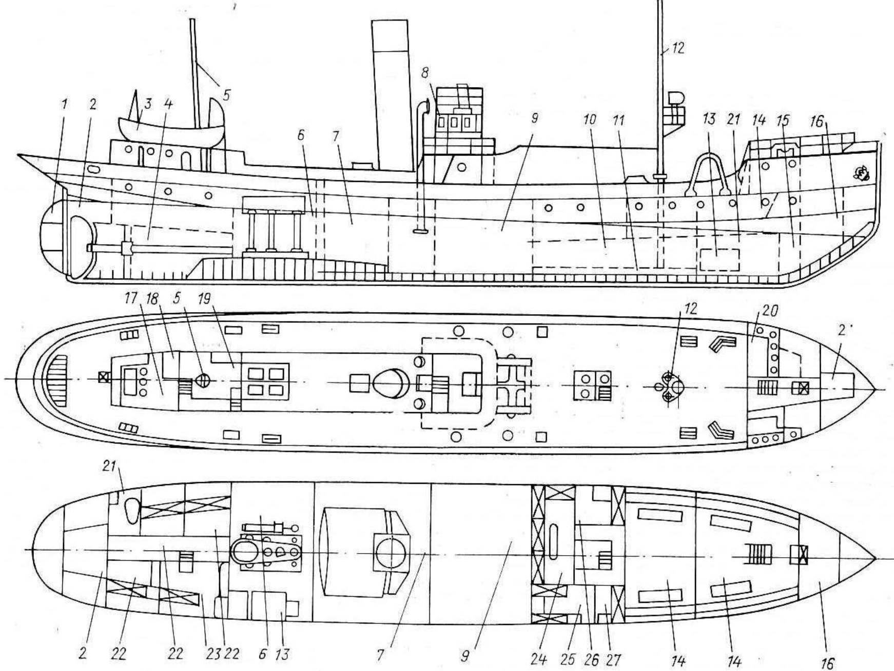
Пароход-тральщик типа «Искра»: а — продольный разрез; б — план верхней палубы; в — план жилой палубы и трюма.
