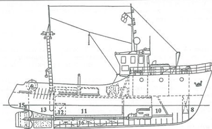
Pokład główny
