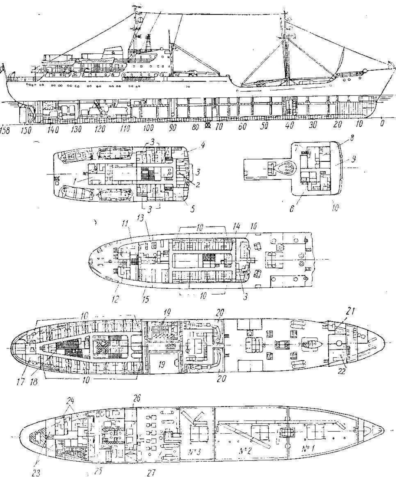
Рис. 206. Общее расположение производственно-транспортного рефрижератора типа «Таврия».
