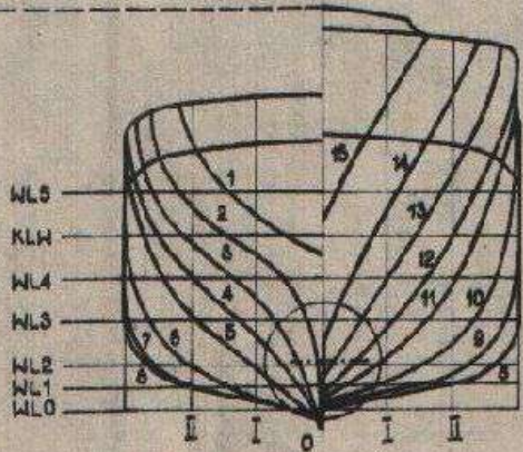
PRZEKROJE POPRZECZNE KADŁUBA
