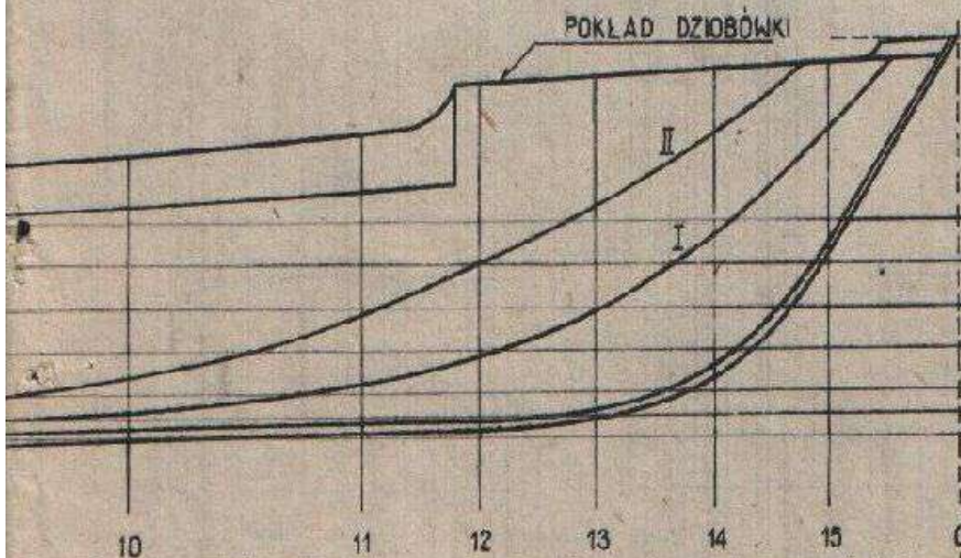
NADBURCIE POKLAD GŁÓWNY POKLAD DZIÓBÓWKI
