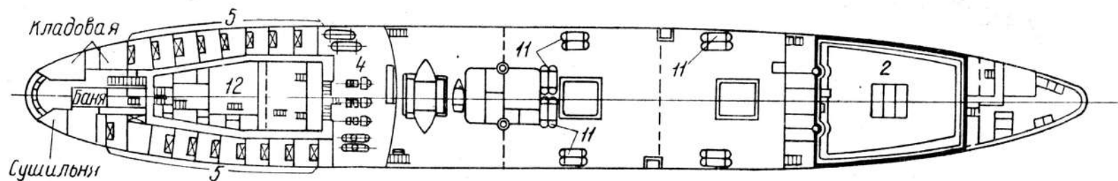
Рис. 75. Общее расположение транспортного рефрижератора типа «Сибирь».
