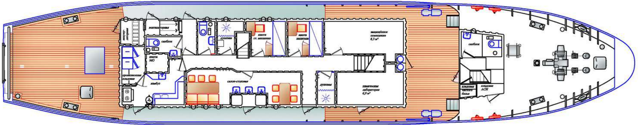
Верхняя палуба
