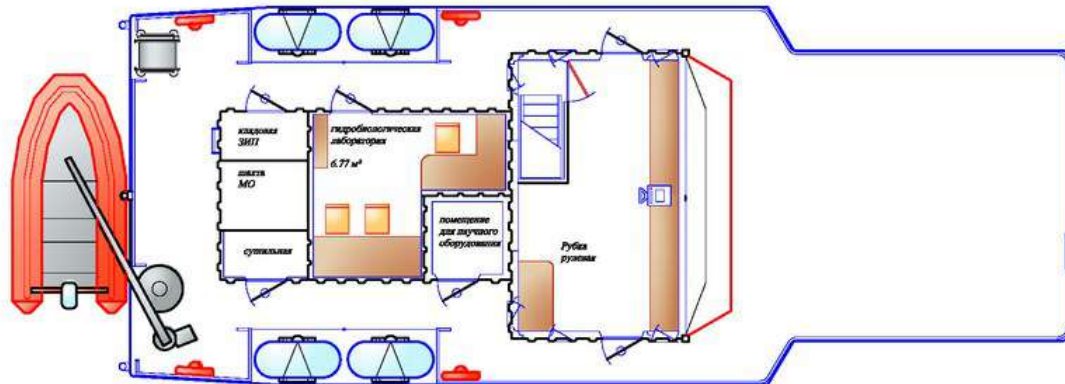
Рубка 2 яруса
